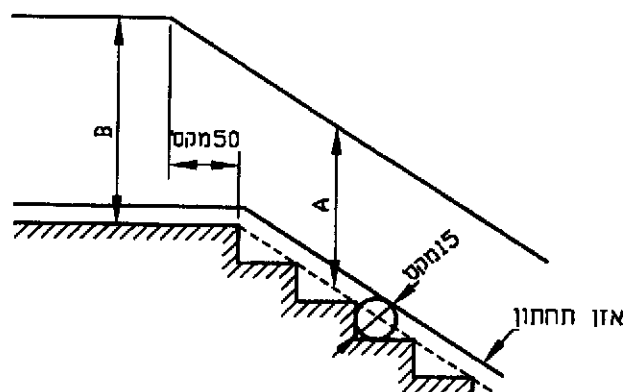
צויר 6 (סכמתי בלבד) (המידות בסנטימטרים)
