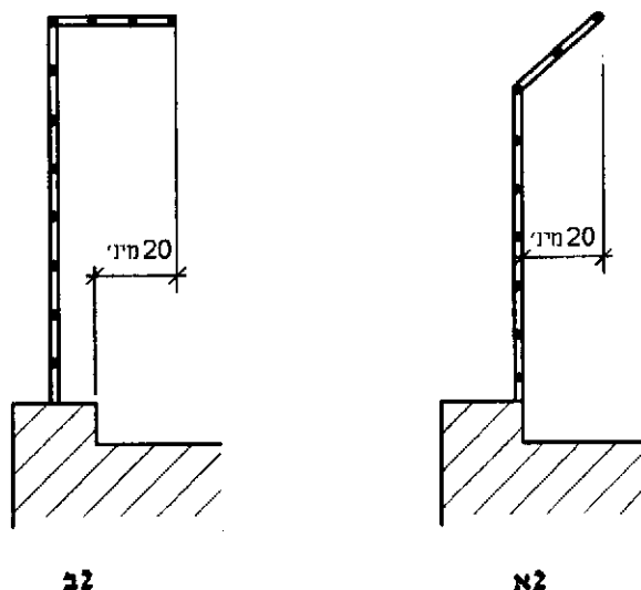
צירור 2 (סכמתי בלבד) (המידות בסנטימטרים)
