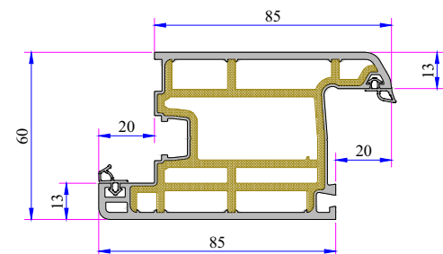
Door Sash Profile
